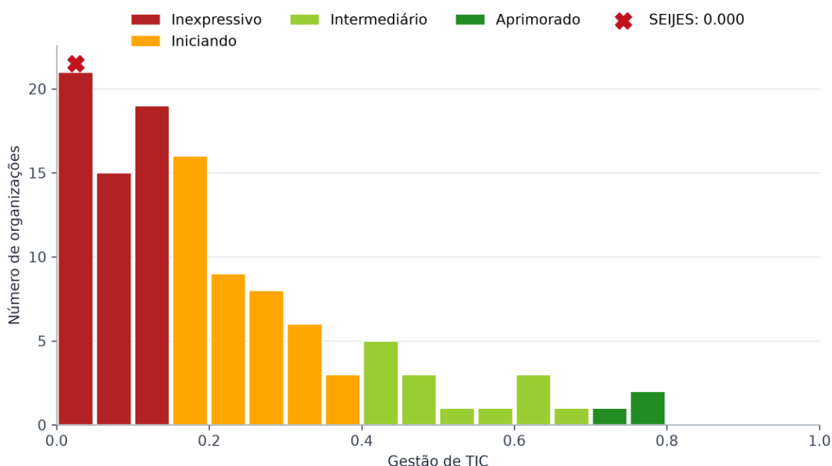
Figura 7 - Resultado do componente Gestão de TIC da organização SEIJES
