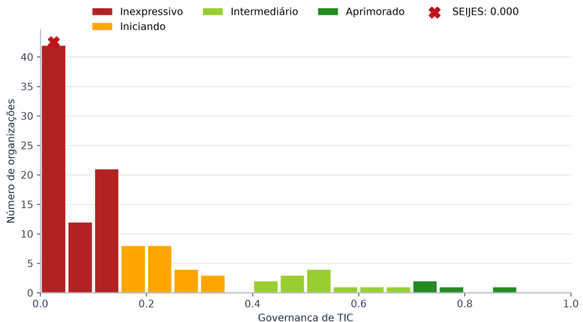
Figura 6 - Resultado do componente Governança de TIC da organização SEIJES
