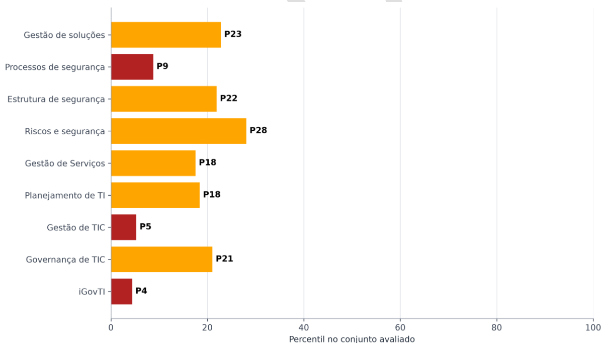
Figura 14 - Comparação da posição relativa da organização SEIJES nos indicadores avaliados
