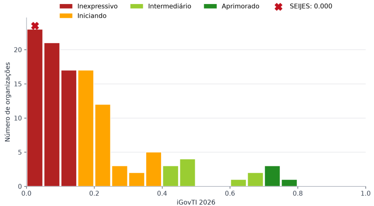
Figura 4 - Distribuição dos resultados do iGovTI 2026 e posição da organização SEIJES
