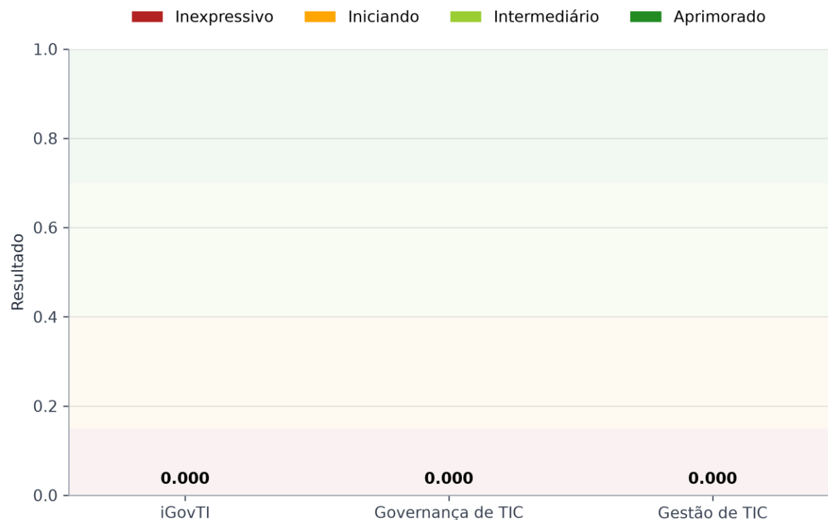
Figura 5 - Resultado da organização SEIJES por componentes do iGovTI 2026
